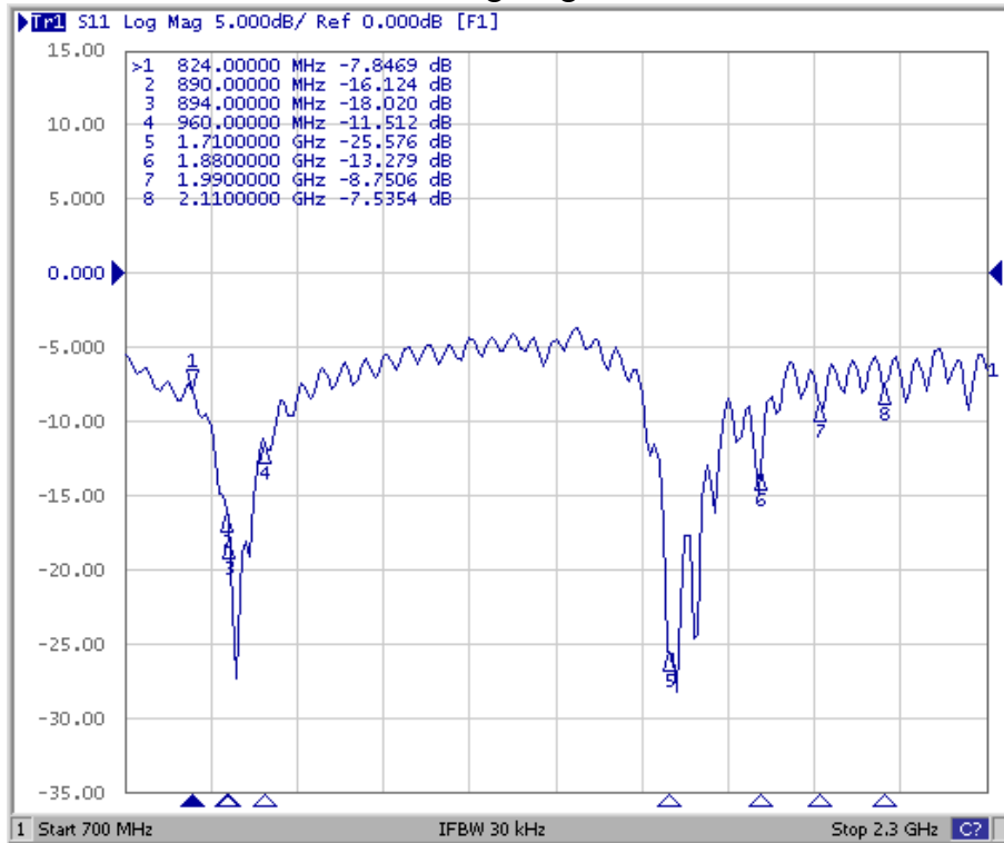
Log Mag
