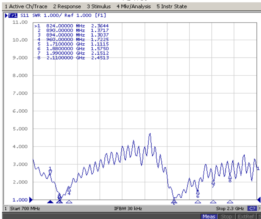
VSWR
